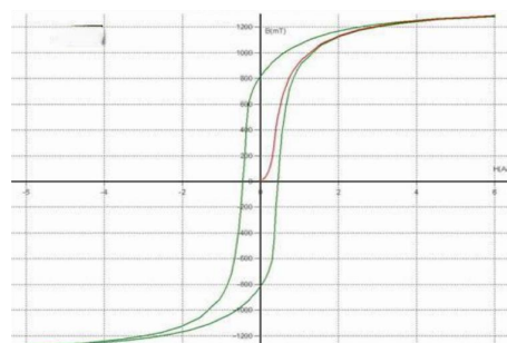
1K107B B-H Loop
